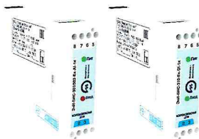
Рисунок 2 — Внешний вид барьеров серии ЭНИ-БИС-3xx-Ex
